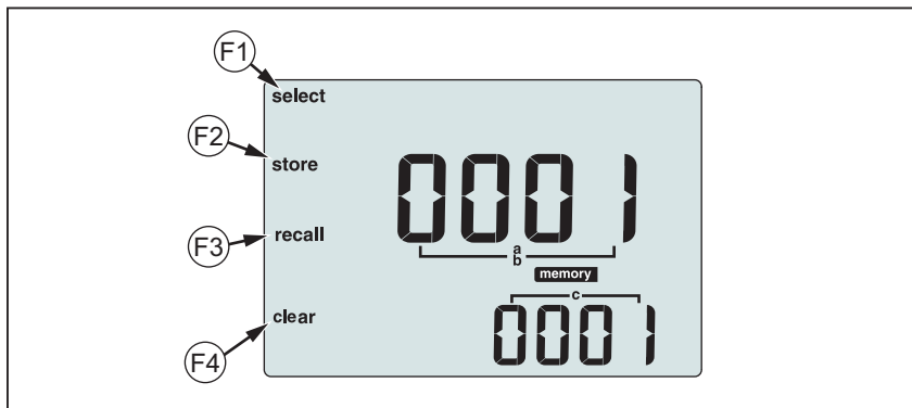
Afbeelding 15. Geheugenmodus
