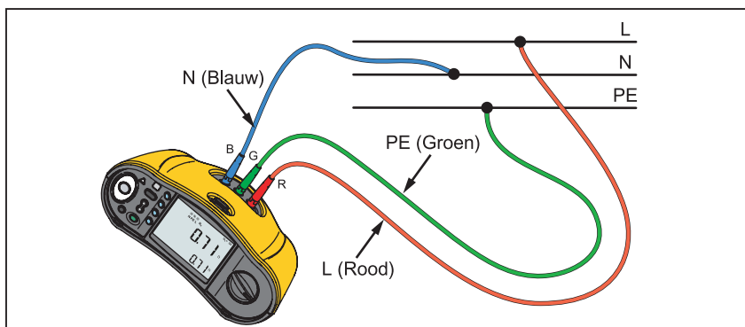
Afbeelding 13. 3-draads aansluiting voor lustest van aardingsweerstand (no-trip-modus)
