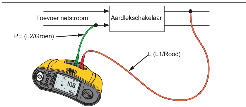
Afbeelding 8. Aansluiting voor de test van aardlekschakelaars op elektrische IT-systemen
