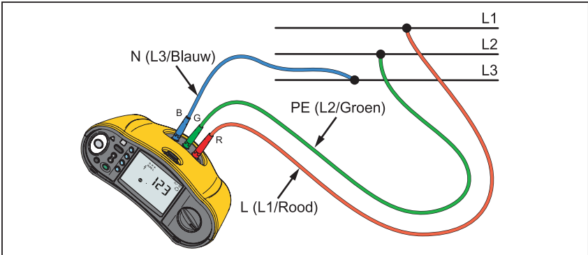
Afbeelding 10. Aansluiting voor faserotatietest
