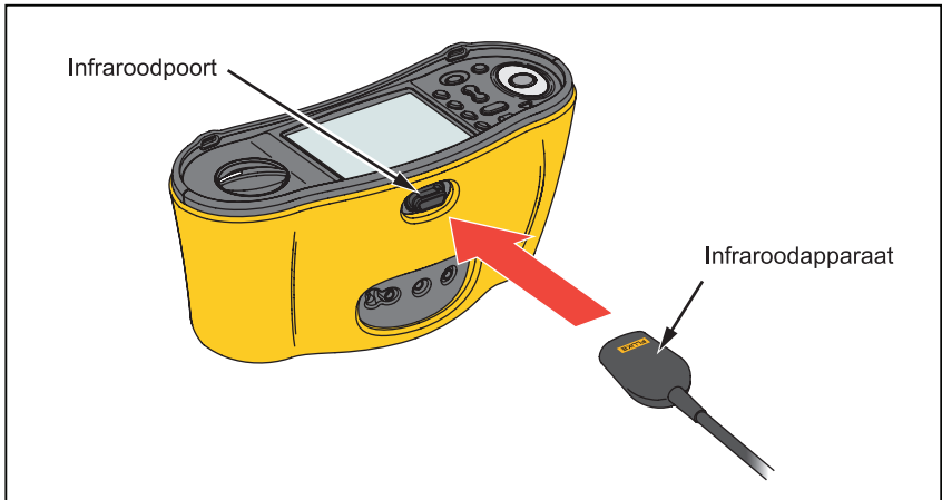
Afbeelding 16. Seriële IR-kabel bevestigen
