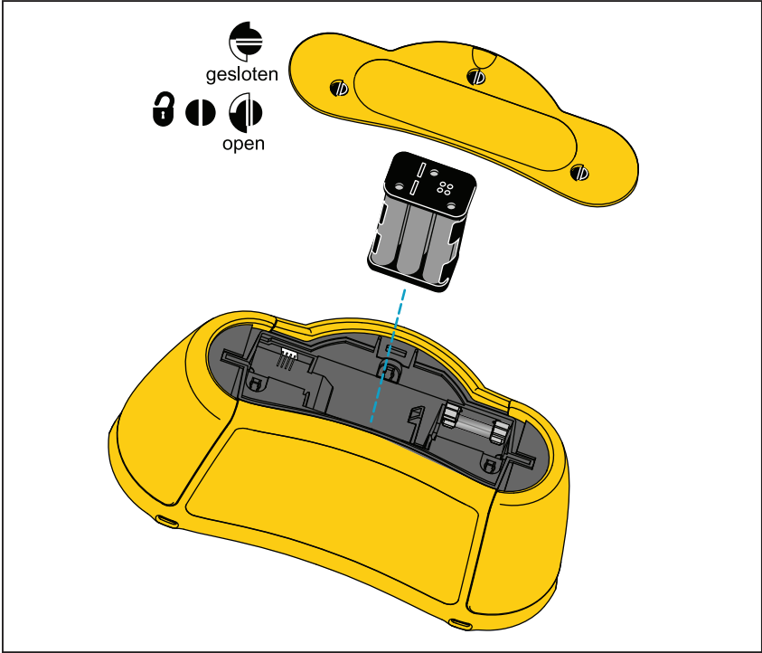
Afbeelding 17. Batterijen vervangen
