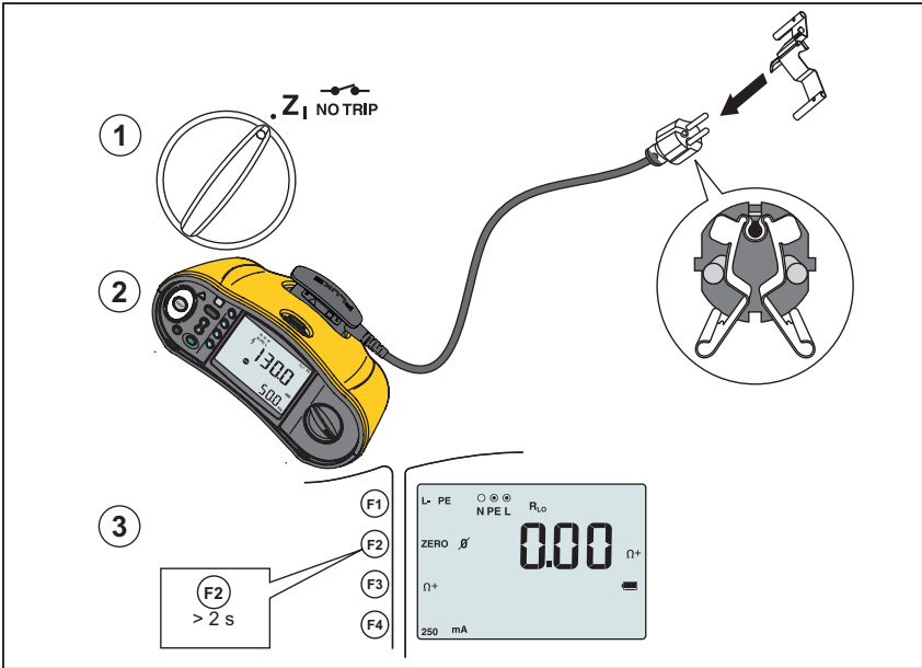
Afbeelding 2. Nulsteldisplay
