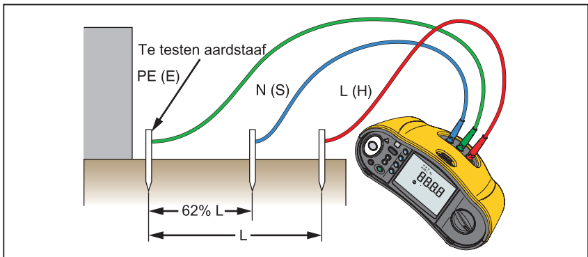
Afbeelding 12. Aansluiting voor aardingsweerstandtest
