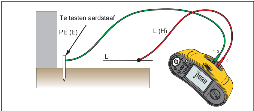
Afbeelding 14. 2-draads aansluiting voor lustest van aardingsweerstand (hogestroom-tripmodus)
