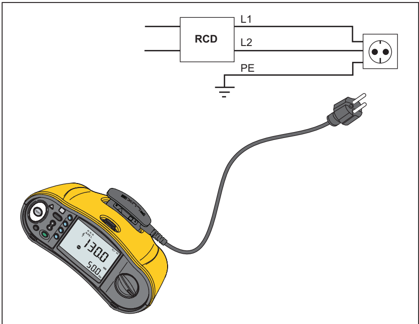
Afbeelding 9. Configuratie met enkel meetsnoer
